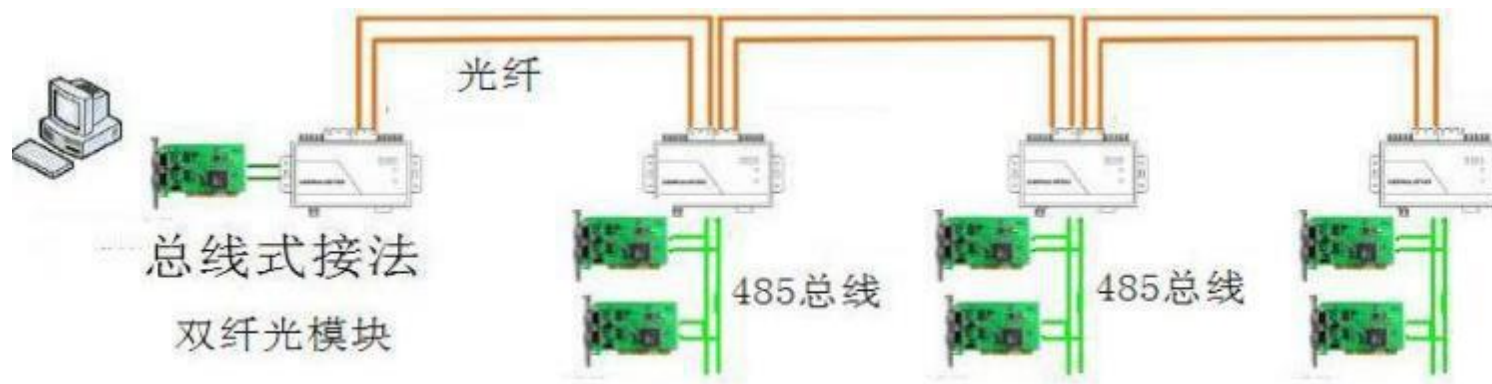
图 1 双纤总线式接法
