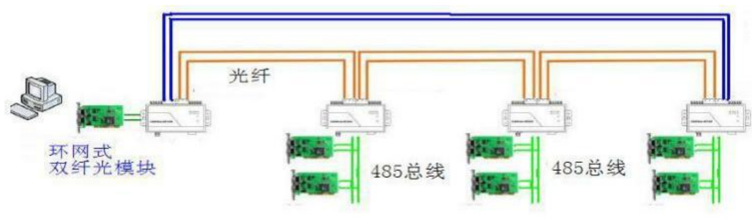
图 3 双纤环网式
