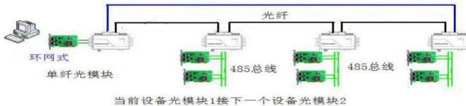
图 4 单纤环网式
